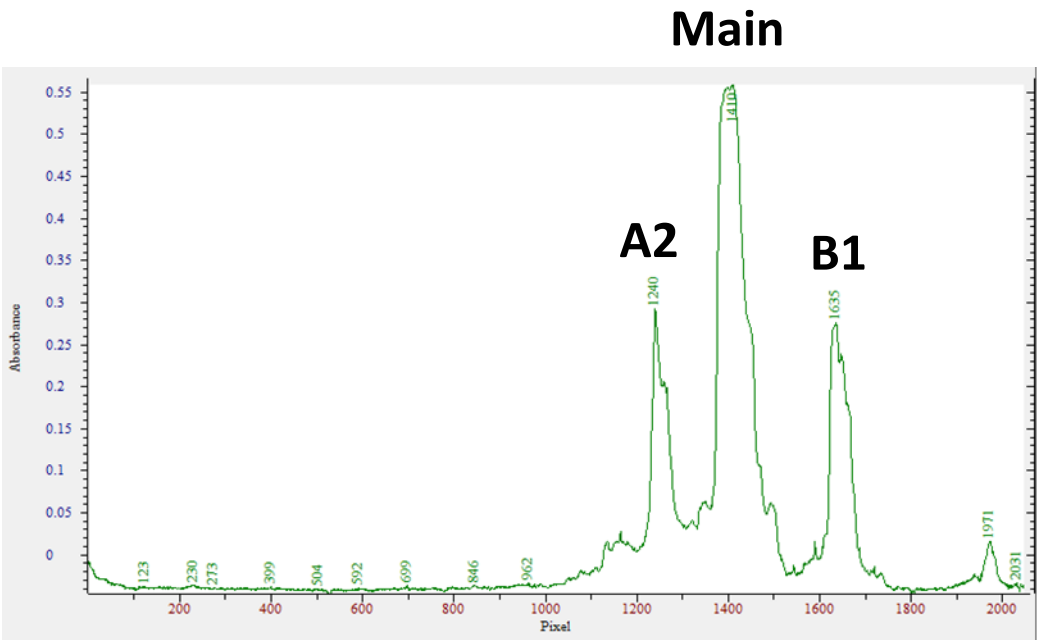
Mab iCIEF profile in preparative mode
